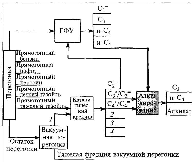
Рис. 8.3. Процессы нефтепереработки.
