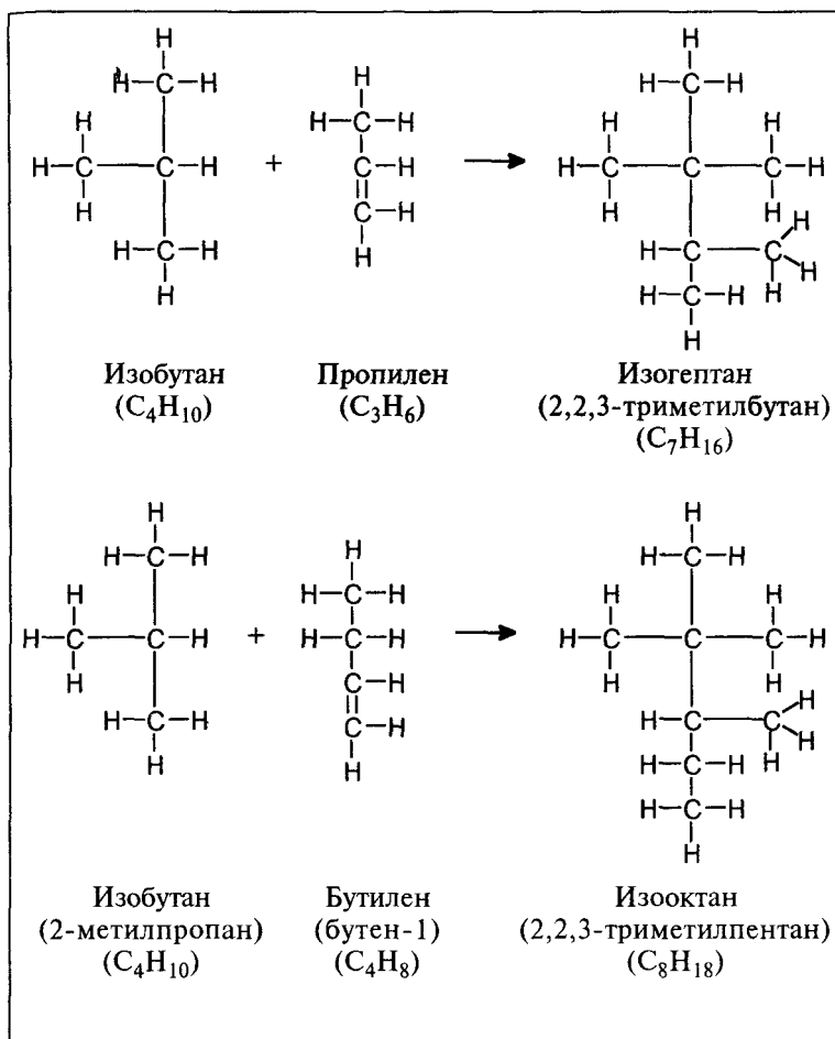
Рис. 8.1. Алкилирование пропилена и бутилена (бутена-1).
