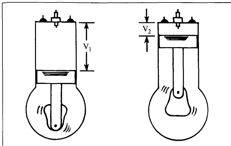
Рис. 12.2. Степень сжатия — это V_1/V_2 .
