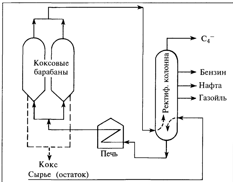
Рис. 10.3. Коксование.
