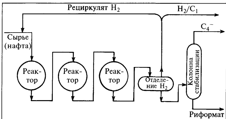
Рис. 9.2. Каталитический риформинг.
