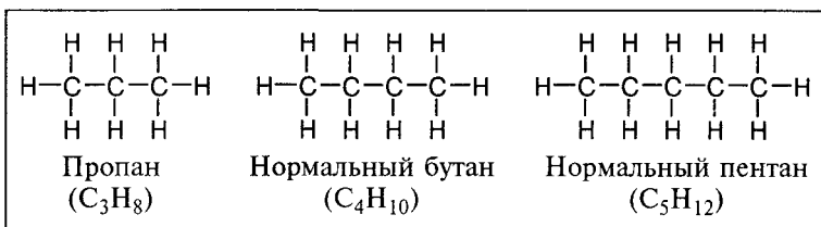
Рис. 5.3. Пропан, нормальный бутан и нормальный пентан.
